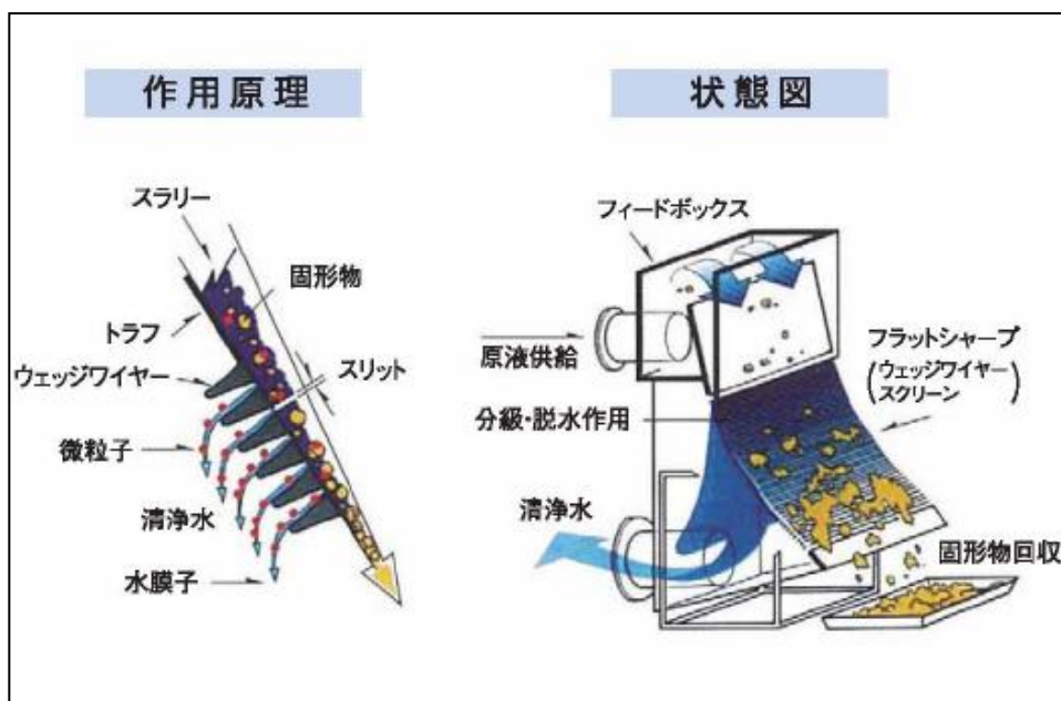
作用原理図
